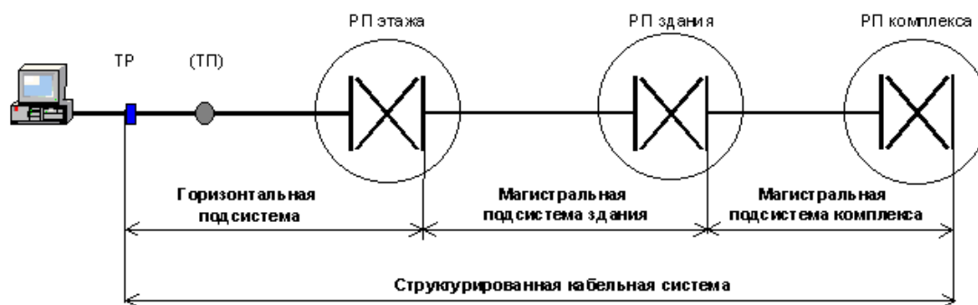
Рис. 1. Подсистемы СКС
