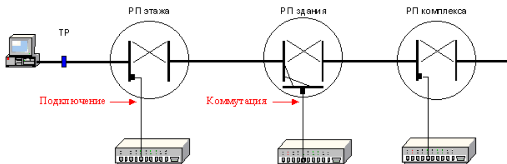
Рис. 3. Интерфейсы СКС
